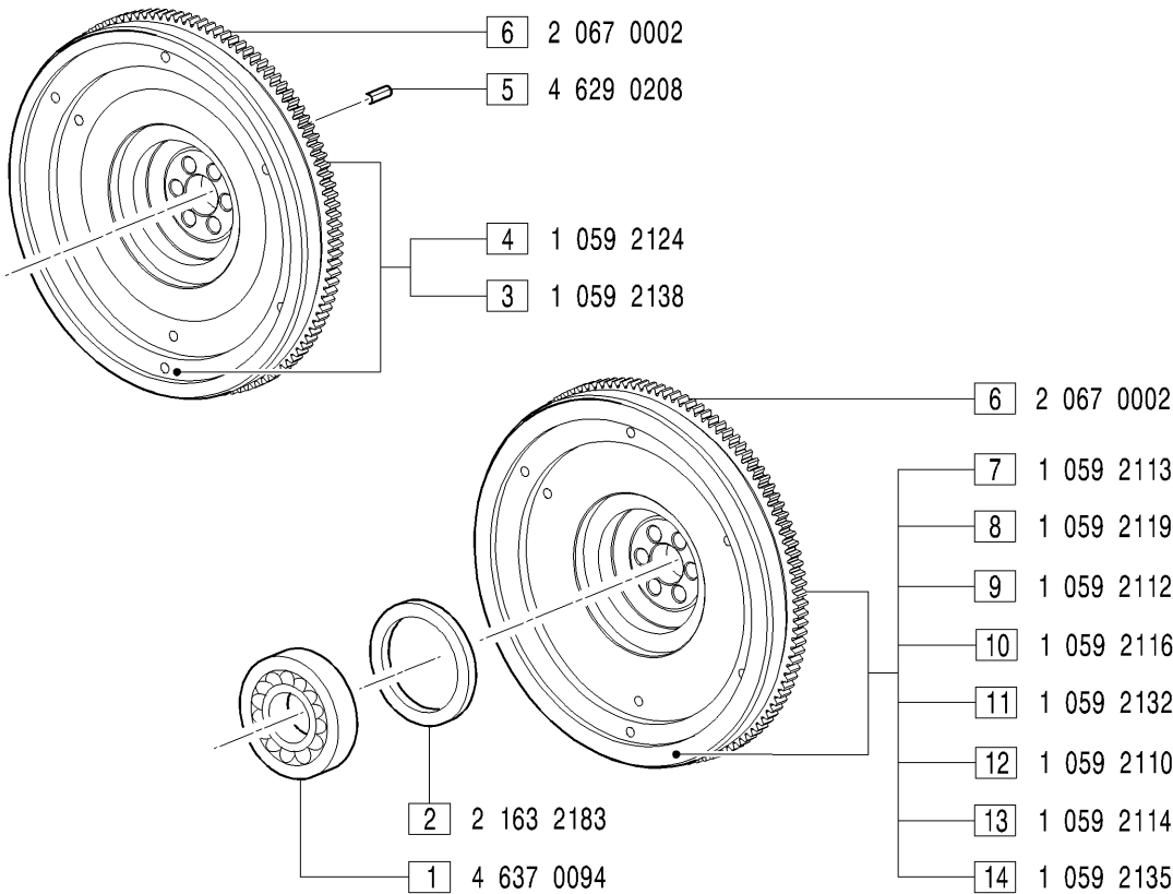
GRUPPI VOLANI - Flywheels groups
