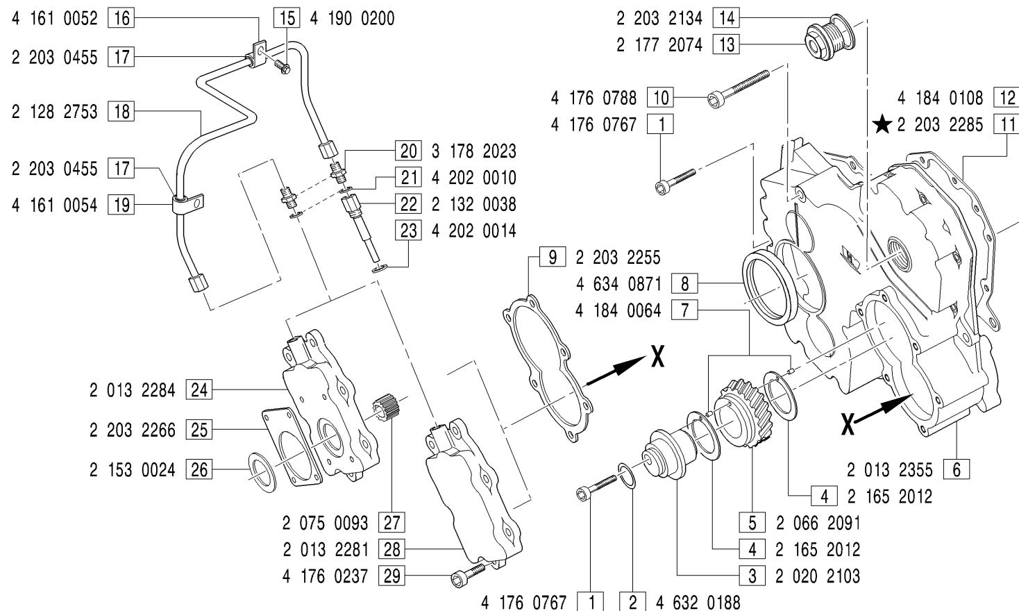
GRUPPI COPERCHIO ANTERIORE - Front cover groups
