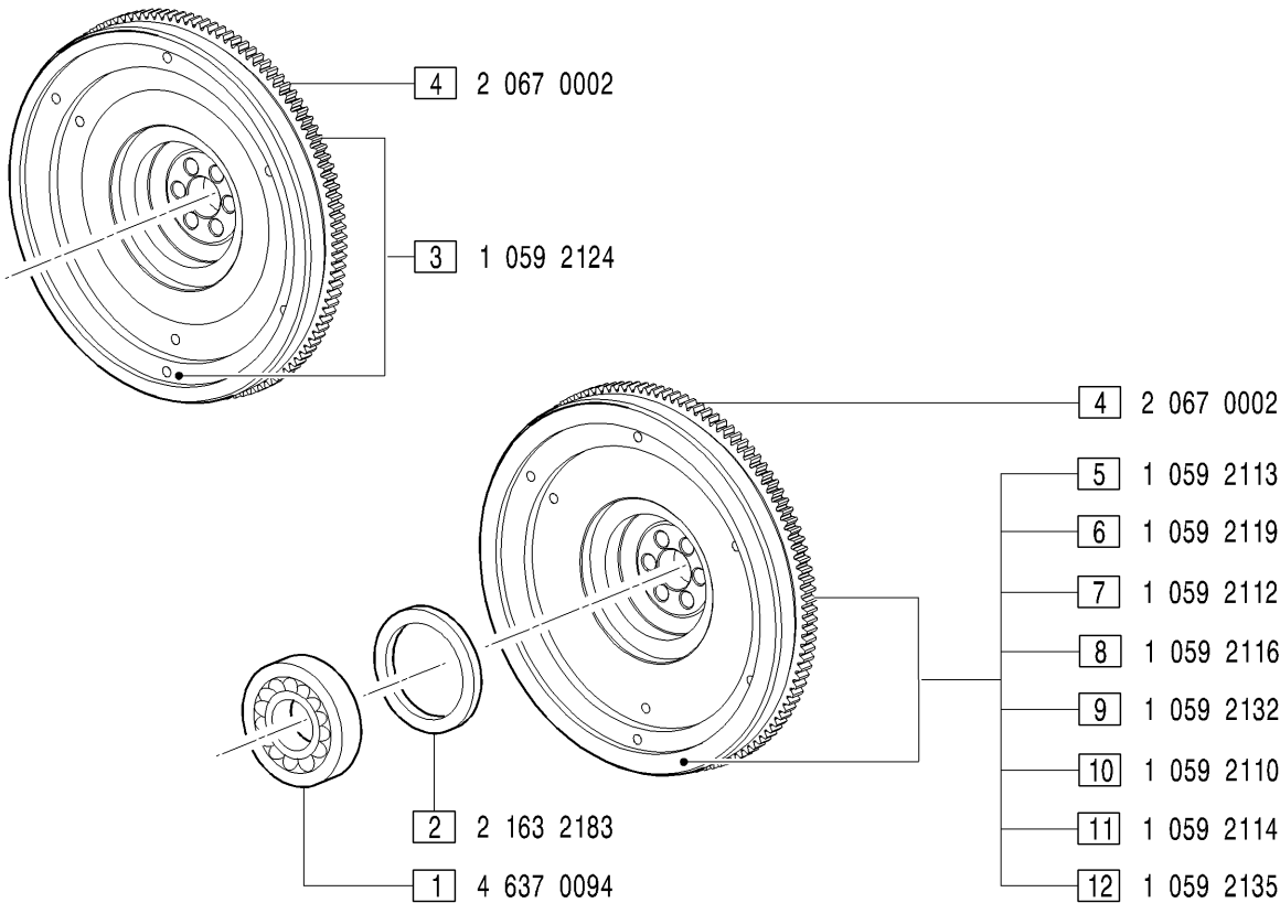
GRUPPI VOLANI - Flywheels groups
