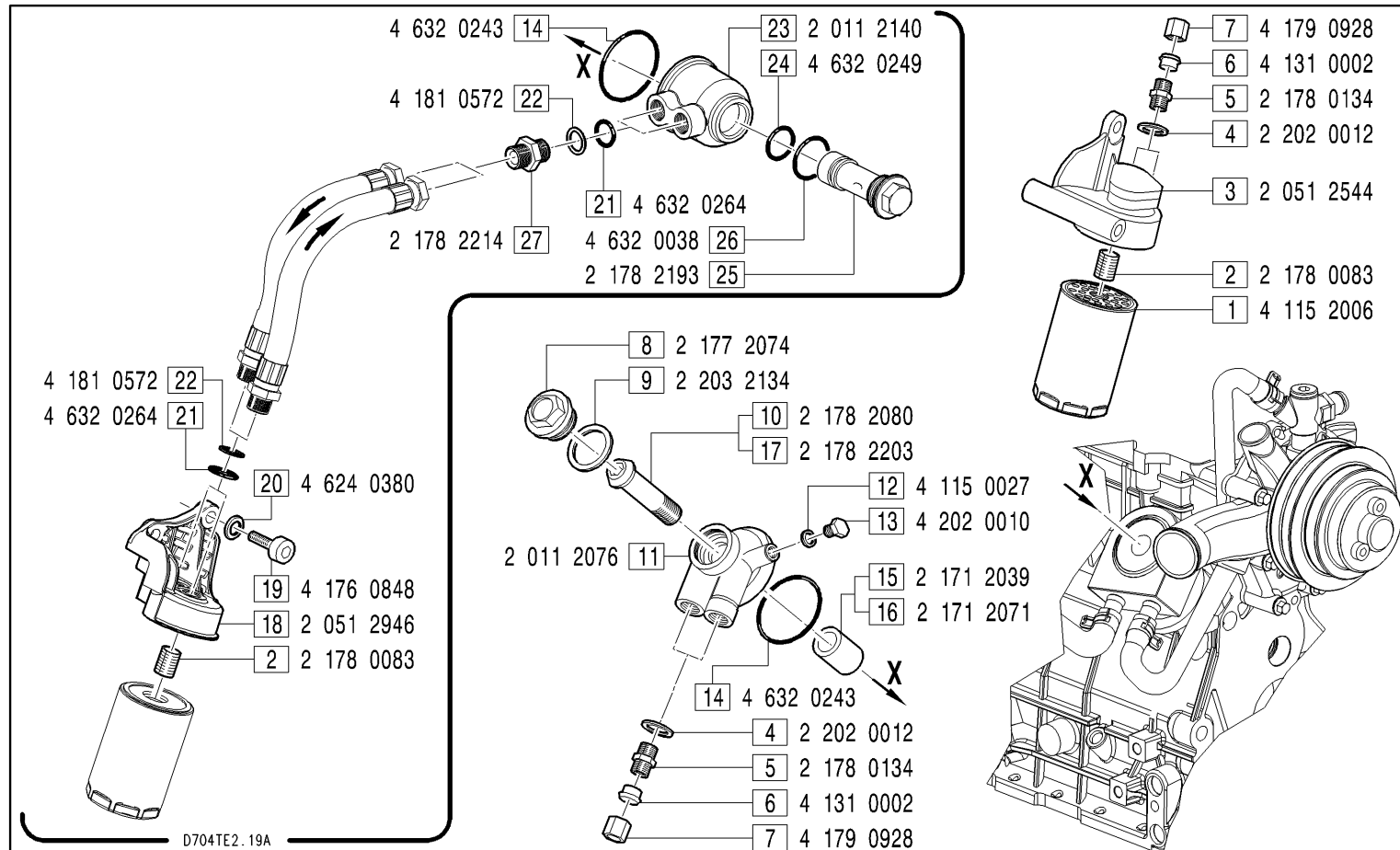
GRUPPO FILTRO OLIO A DISTANZA- Remote oil filter group
