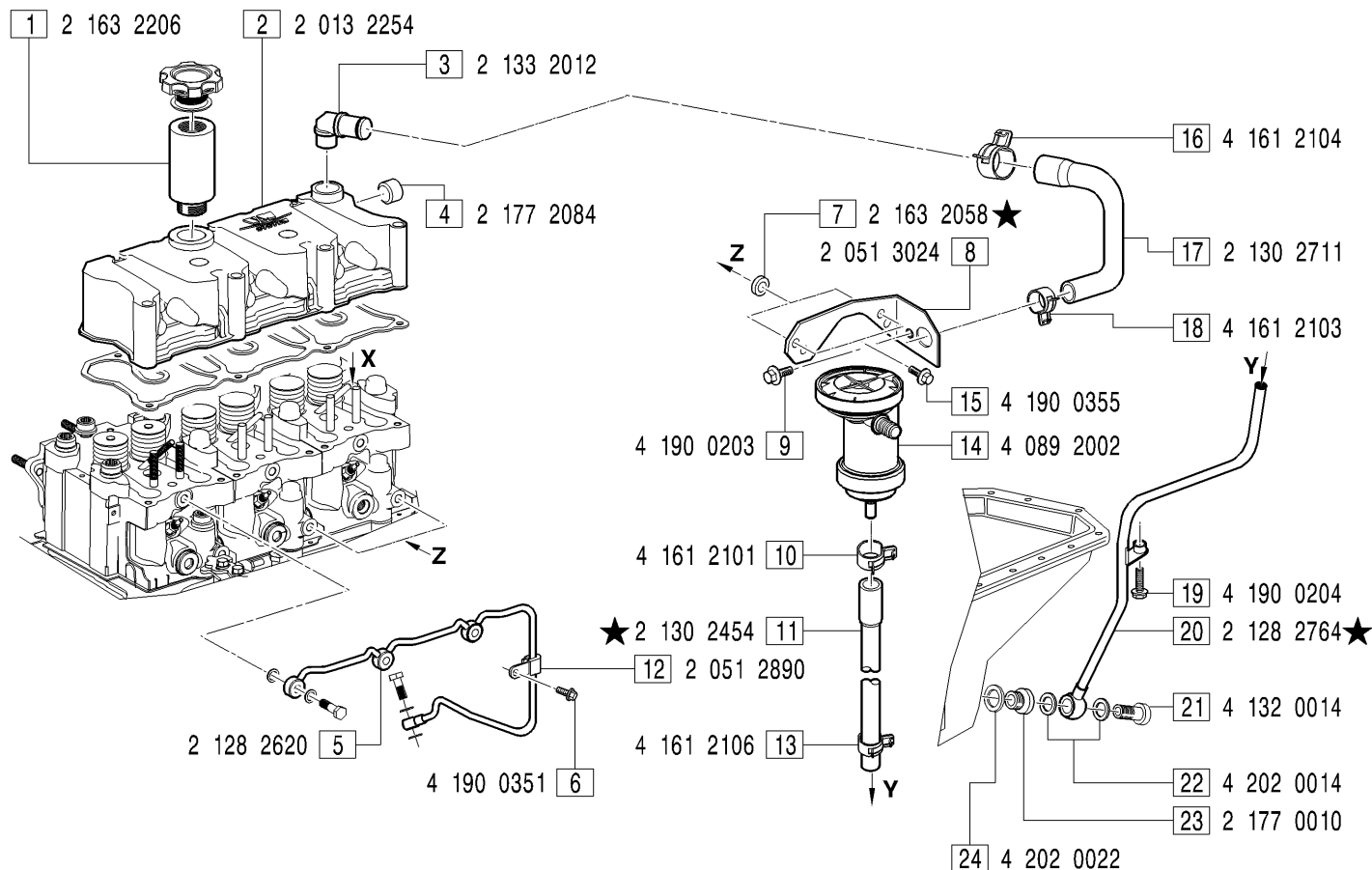
GRUPPI COPERCHI BILANCIERI - Rocher arm covers groups
