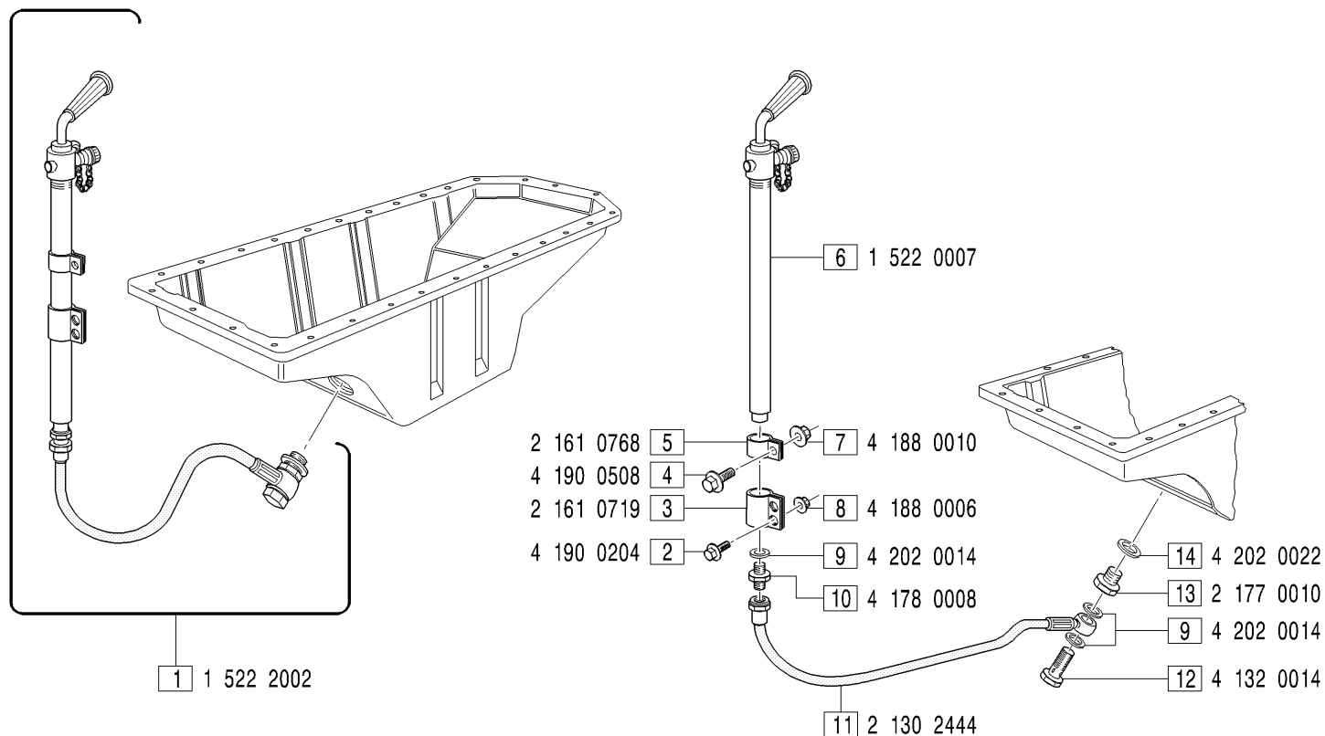
GRUPPO POMPA ESTRAZIONE OLIO - Oil scavage pump group
