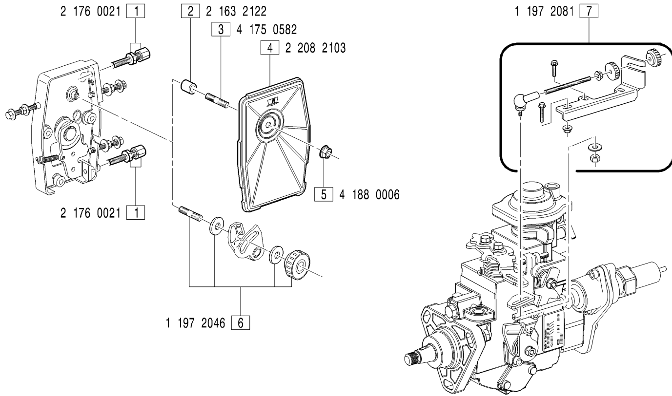
GRUPPI PROTEZIONE REGOLATORE E COMANDO ACCELERATORE - Governor protection kit and accelerator control groups
