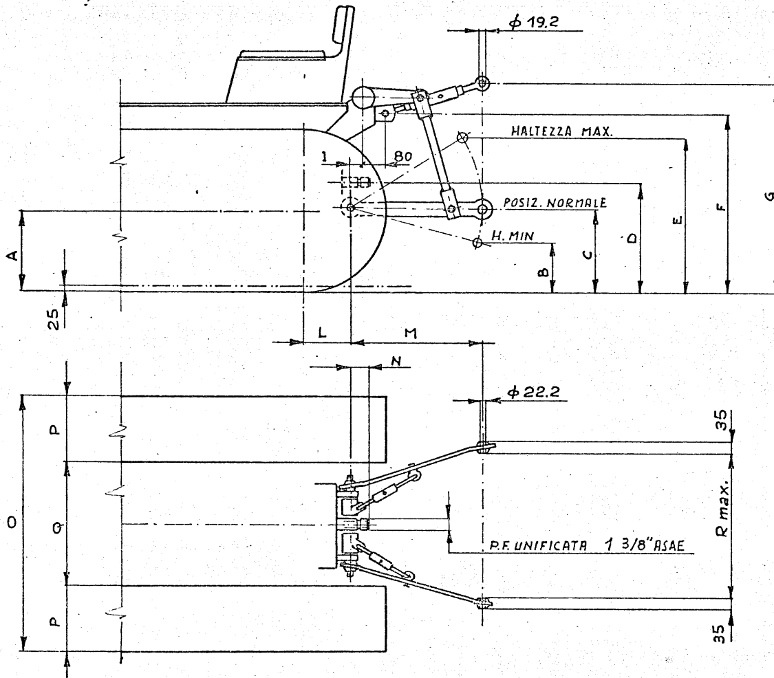
TRATTRICE TIPO
